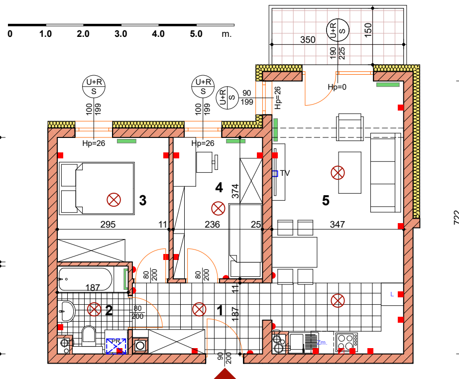
PIĘTRO III
