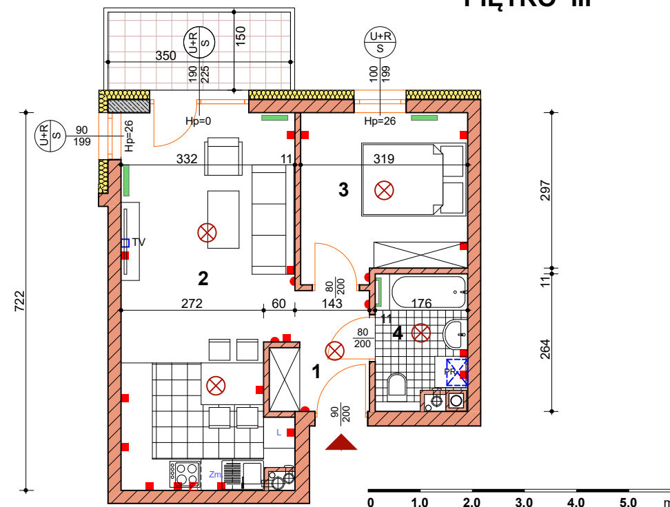
PIĘTRO III
