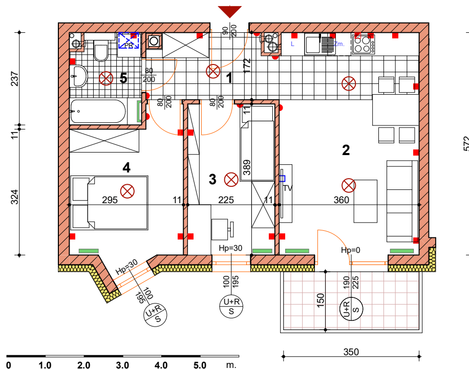
BUDYNEK nr 3 - piętro IV
