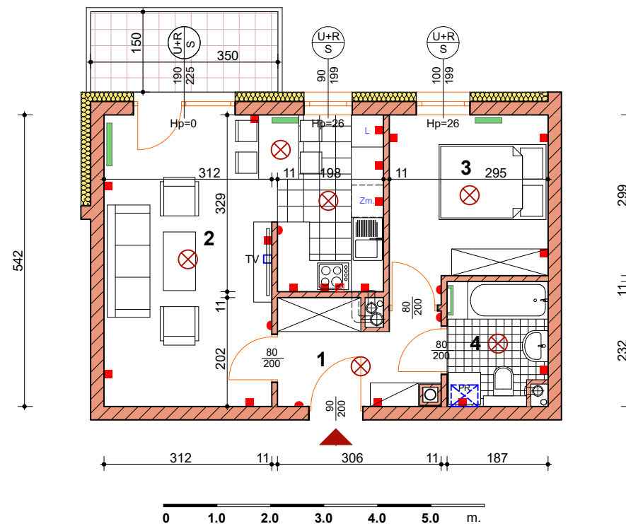
BUDYNEK nr 3 - piętro III
