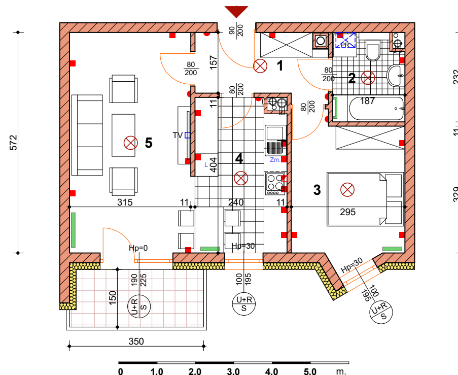
BUDYNEK nr 1 - piętro I
