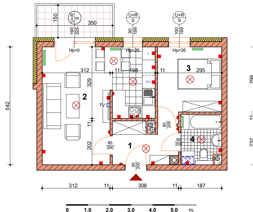
BUDYNEK nr 1 - piętro I
