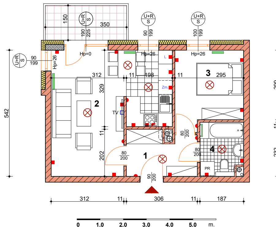
BUDYNEK nr 9 - piętro II
