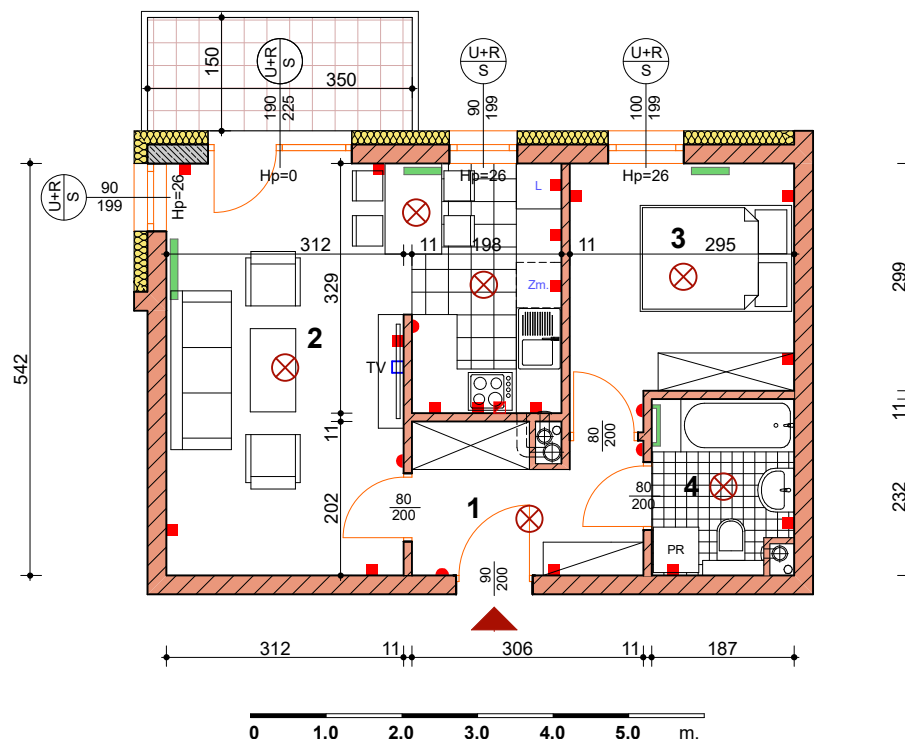
BUDYNEK nr 9 - piętro I
