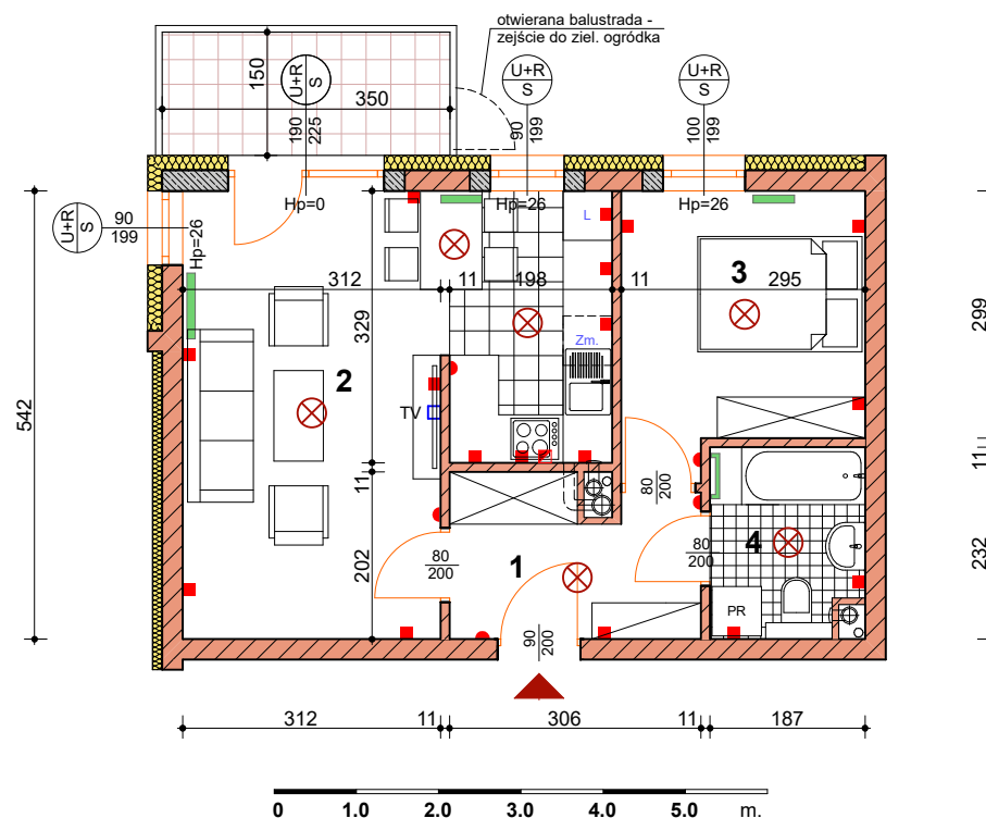
BUDYNEK nr 9 - parter
