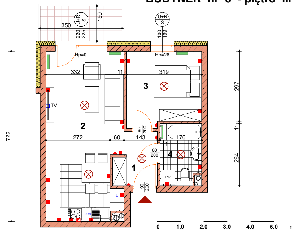
BUDYNEK nr 8 - piętro III
