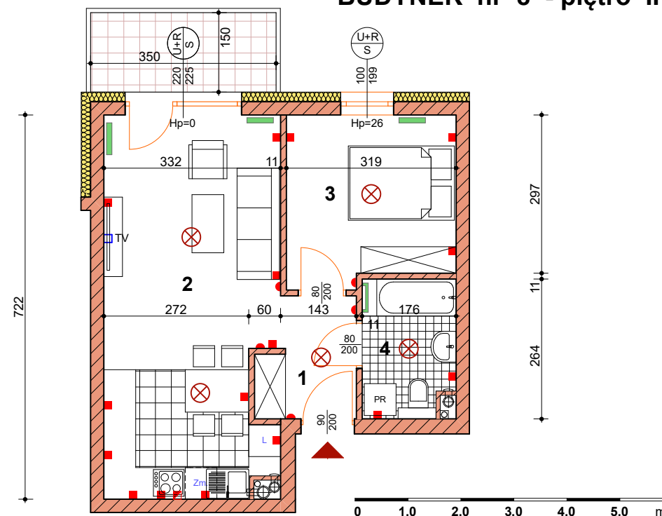
BUDYNEK nr 8 - piętro II
