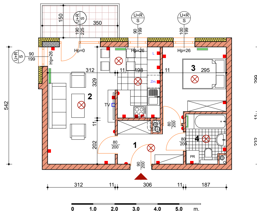
BUDYNEK nr 7 - piętro III
