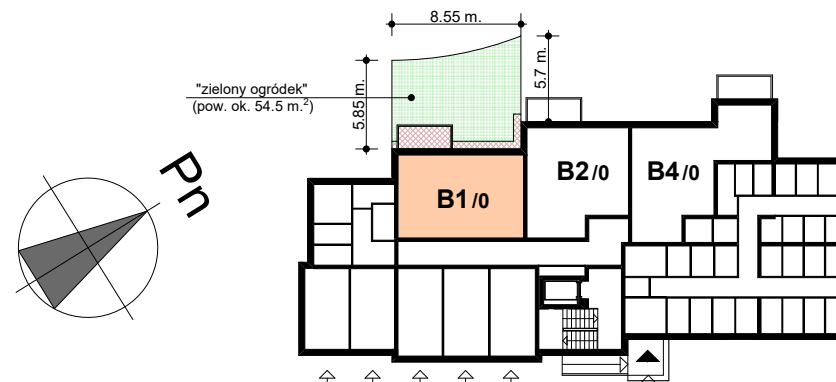
BUDYNEK nr 7 - parter
