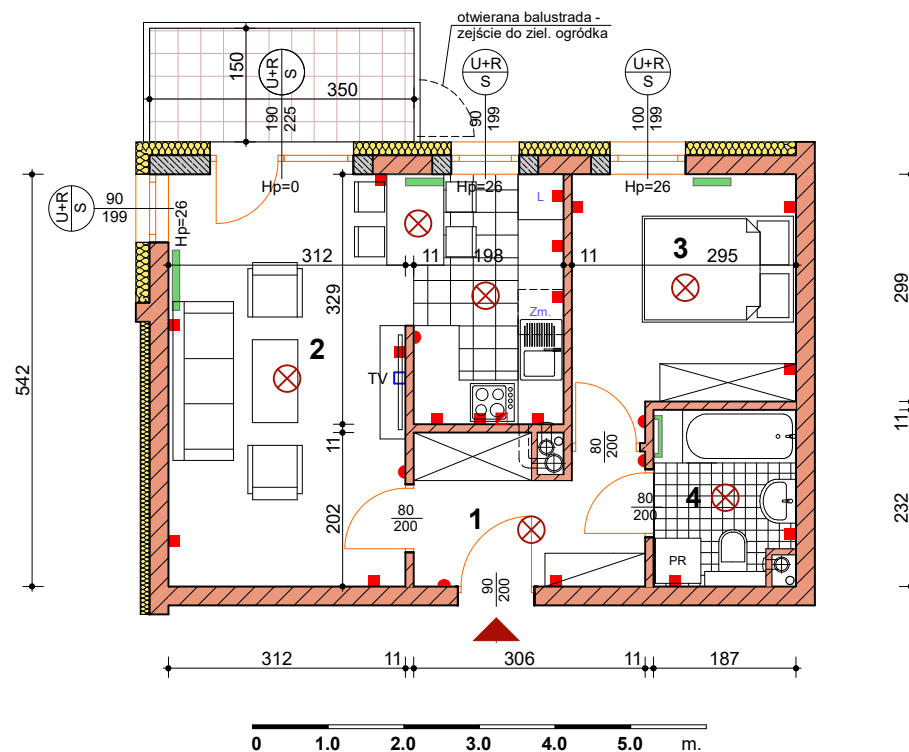
BUDYNEK nr 7 - parter
