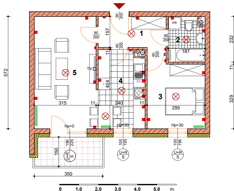
BUDYNEK nr 11 - piętro I
