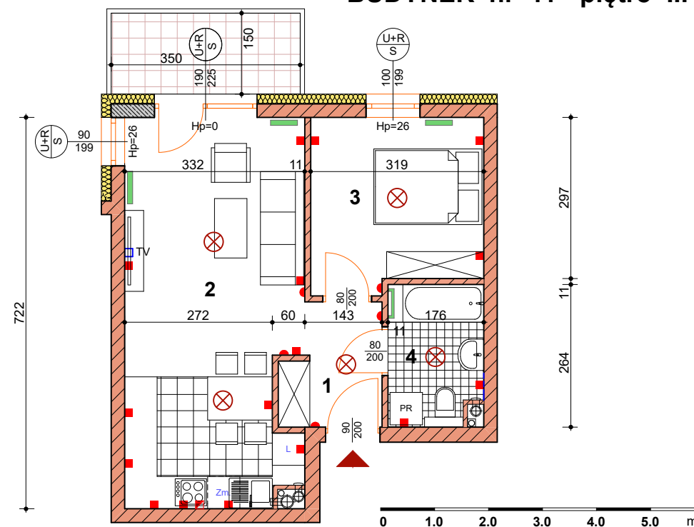
BUDYNEK nr 11 - piętro III
