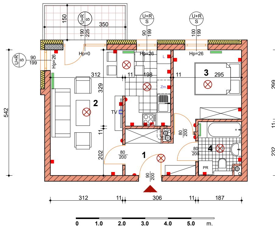
BUDYNEK nr 11 - piętro III
