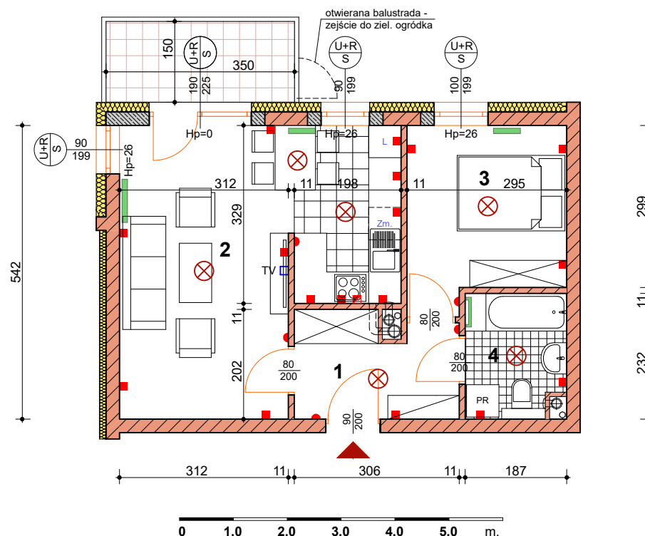
BUDYNEK nr 11 - parter
