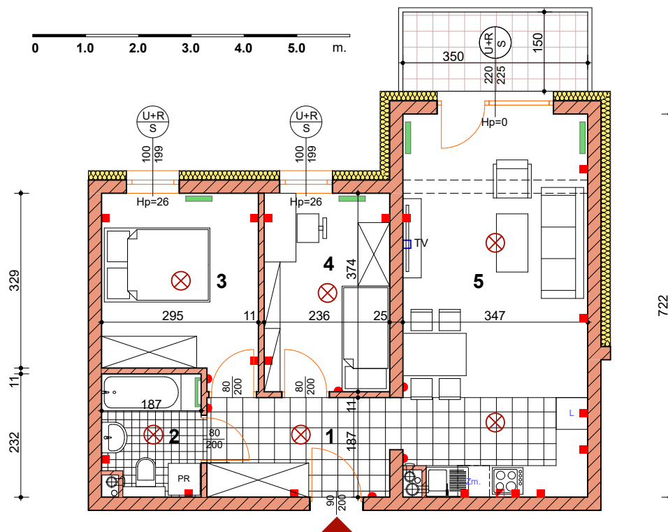
BUDYNEK nr 10 - piętro III
