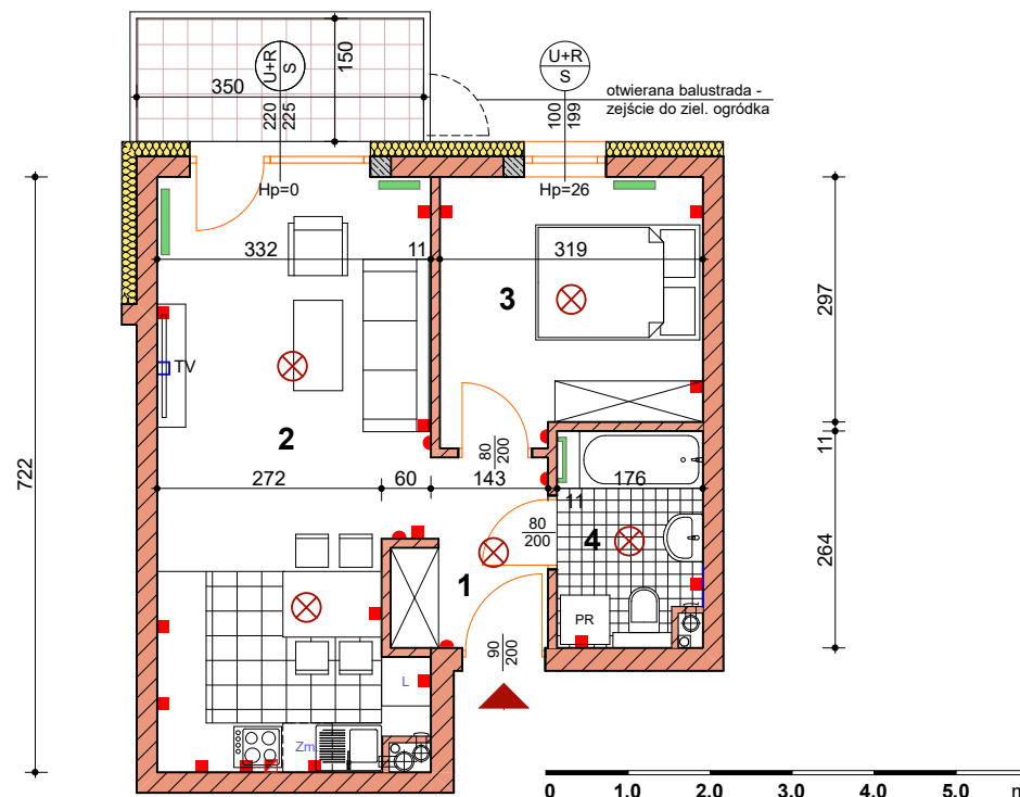
BUDYNEK nr 10 - parter
