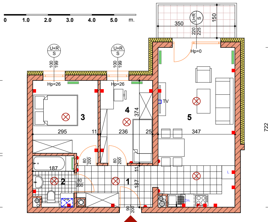
BUDYNEK nr 3 - piętro I
