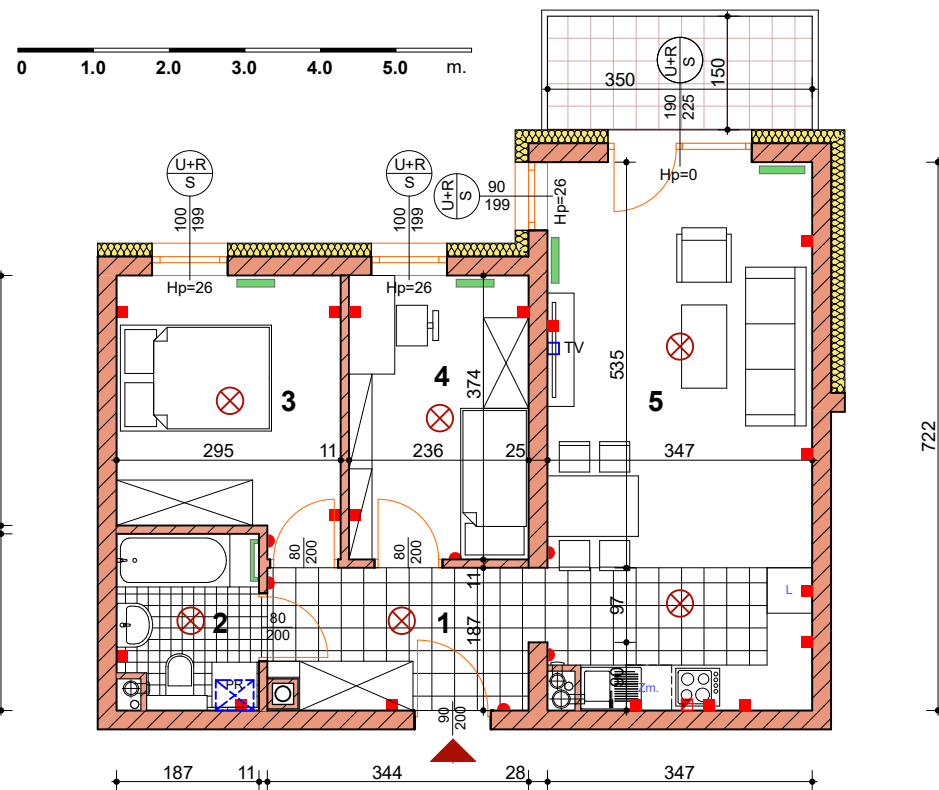
BUDYNEK nr 2 - piętro III
